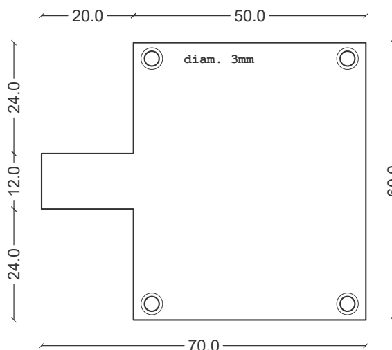
Spessore PCB 1.6mm
